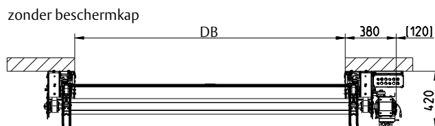
Laserbeschermingsgordijn
